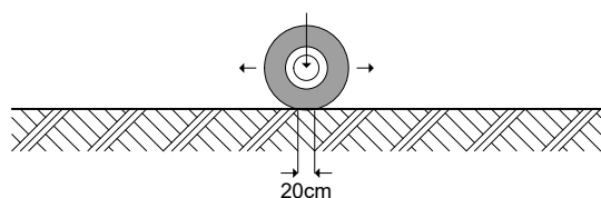
ケース①（頂版上に後輪荷重を載荷する）
