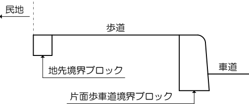
マウンドアップ 歩道 (歩道と車道に段差があります)
