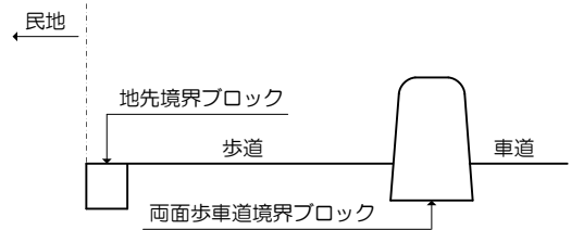
フラット 歩道 (歩道と車道に段差がありません)
